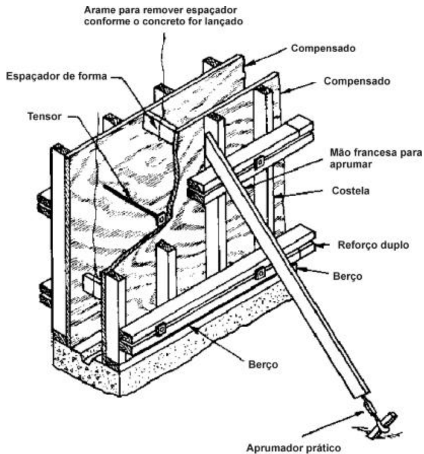
Exemplo de uma parede com aprumador – Aprumador Prático
