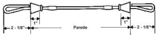
Tensor com laço
